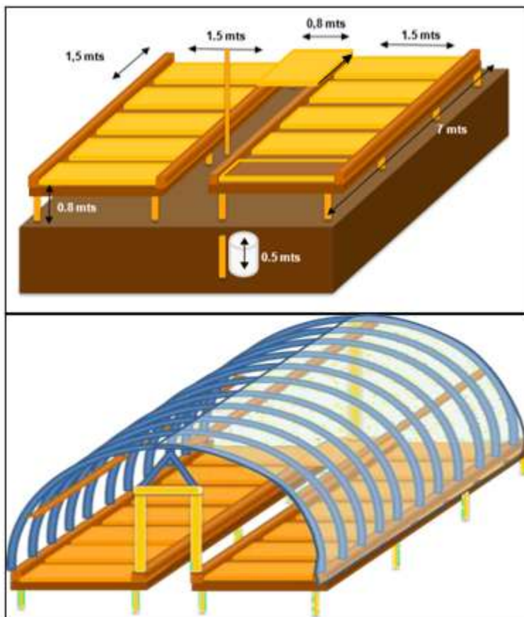
Ilustración 4. Esquema de la Marquesina tipo túnel
