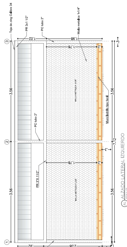
ALZADO POSTERIOR ESCALA 1:5
