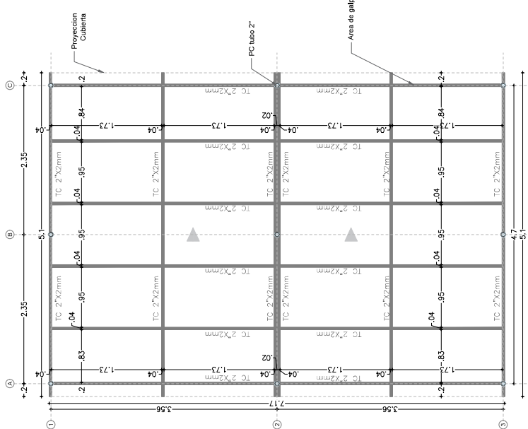
PLANTA ELEMENTOS DE CUBIERTA ESCALA 1:5
