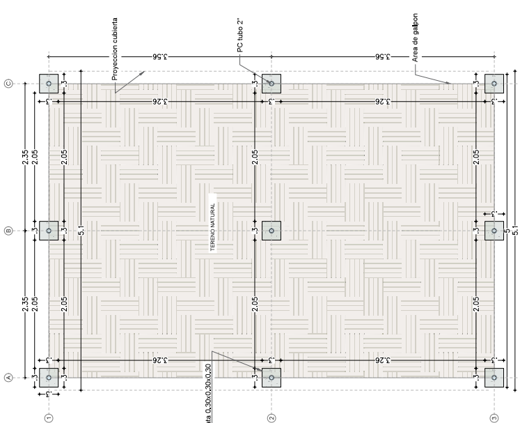
PLANTA DE CIMENTACION ESCALA 1:5
