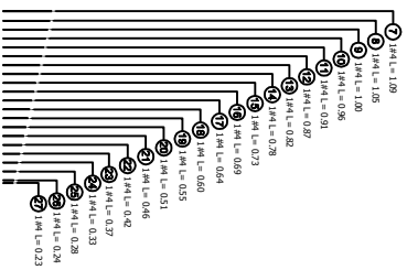
DESPIECE ACERO DE REFUERZO M1 Y M2 EMBARCADERO ESCALA 1/75
