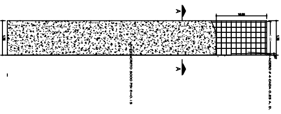
DETALLE EN PLANTA LOSA DE CONTRAPISO ZONA DE BRITES, BASCULA Y PROTECCION
