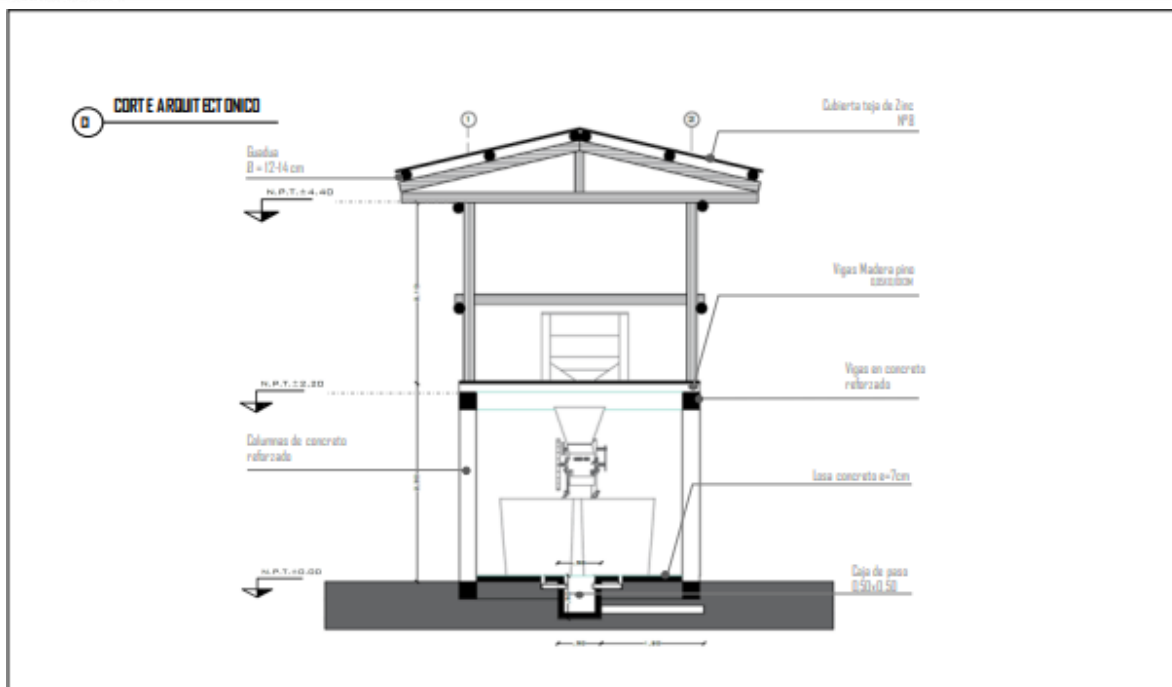
Corte arquitectónico Beneficiadero de café
