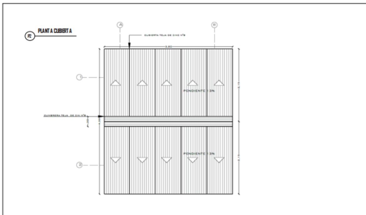
Planta cubierta Beneficiadero de café
