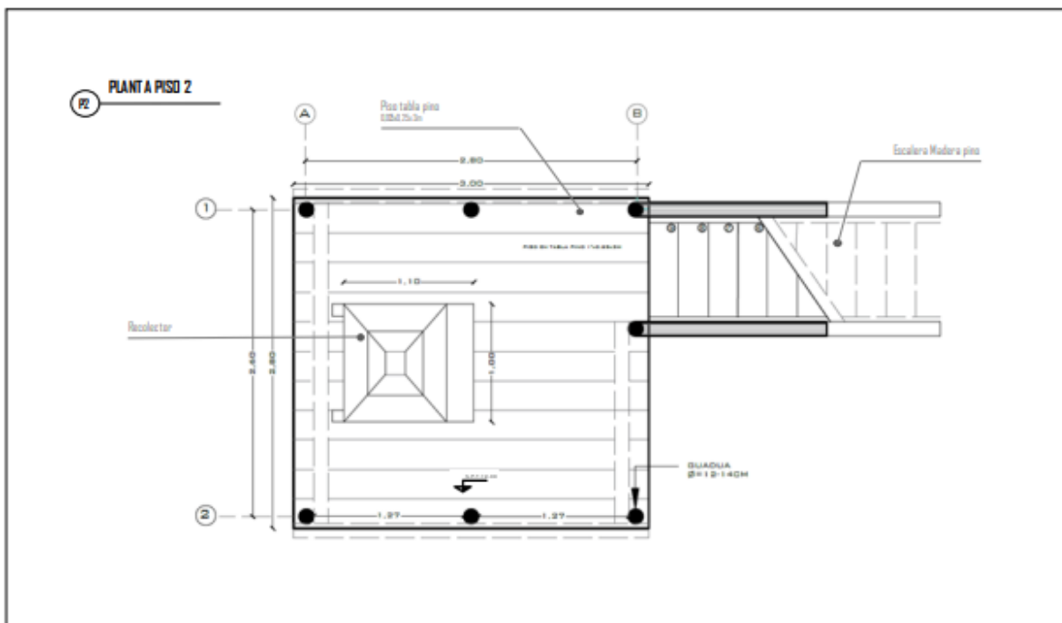
Planta piso 2 Beneficiadero de café
