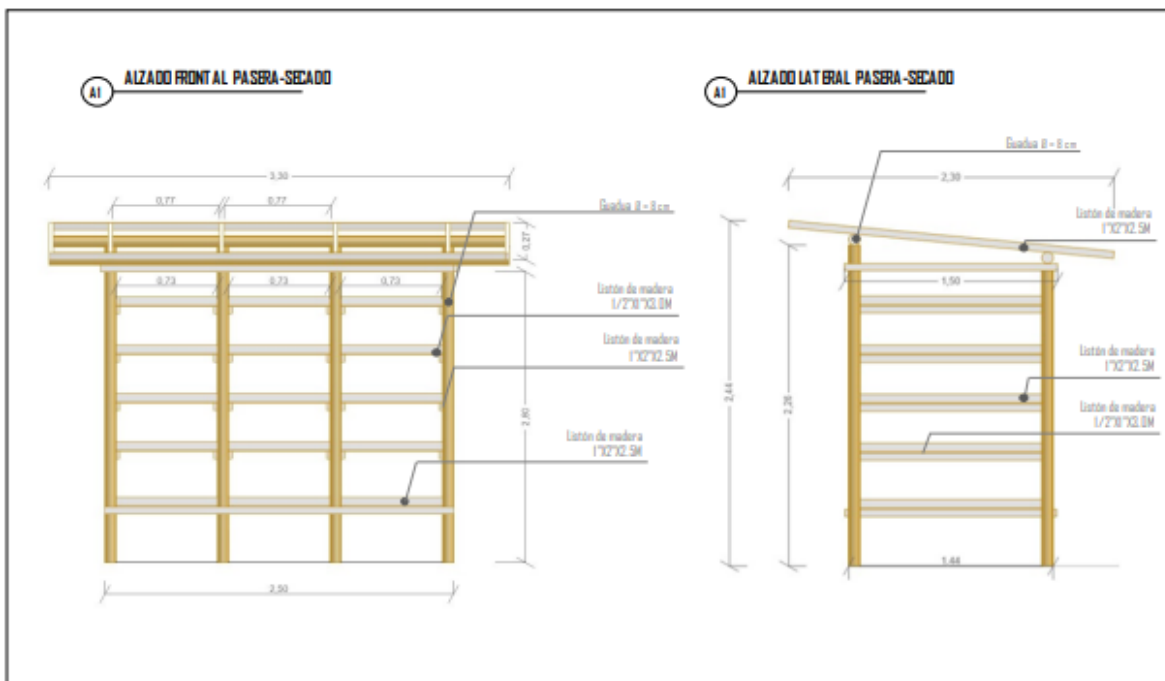
Alzado frontal y lateral Pasera secado de café
