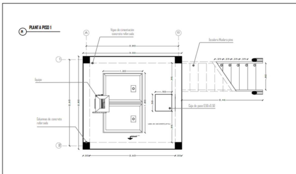
Planta piso 1 Beneficiadero de café
