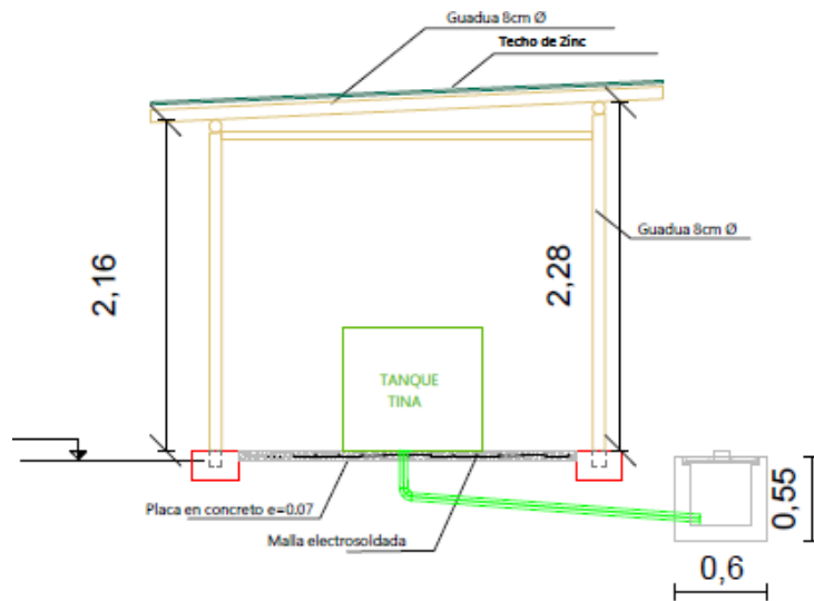
FACHADA LATERAL
