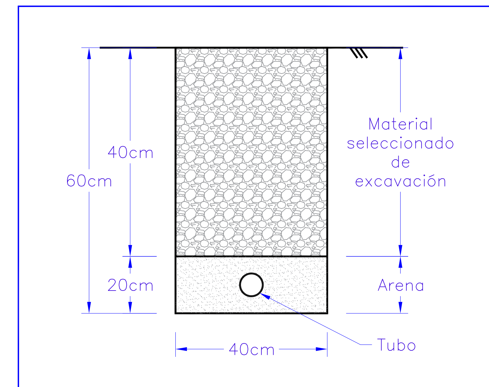
SECCIÓN DE CIMENTACIÓN PARA INSTALACIÓN DE TUBERÍA DE HASTA 4" (medidas en cm)
